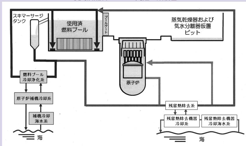
使用済燃料プールの周辺の系統図
