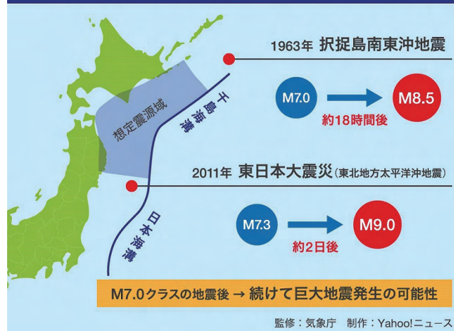
日本海溝・千島海溝の位置／過去の巨大地震
