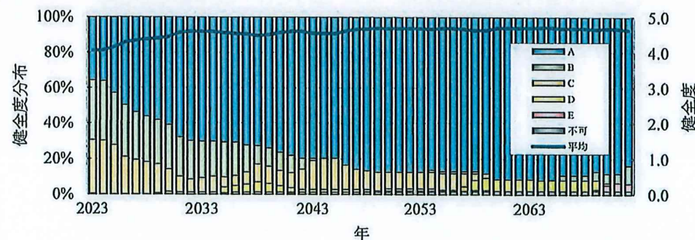
健全度分布の推移 (主部材のみ)
